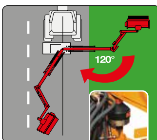
Sistema di massima sicurezza con ritorno automatico tramite accumulatore di azoto (SRA). Hydraulic breakaway with accumulator controlled autorest facility (SRA).
