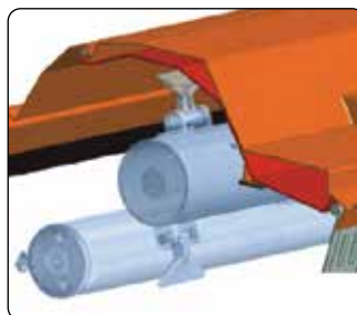
Controltaio interno a protezione integrale del corpo trinciante. Inner lining to fully protect the cutting head.
